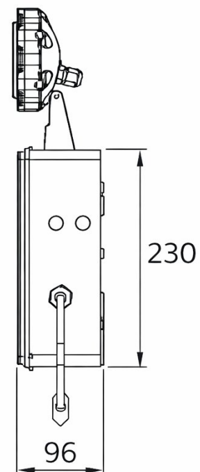
Vista Lateral
